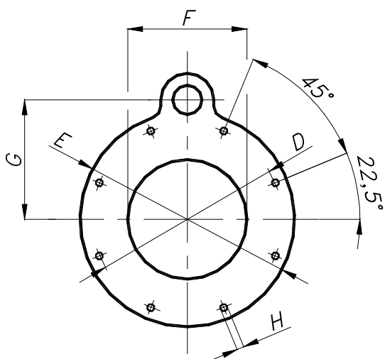
Flange Cosmo 175 - 465
