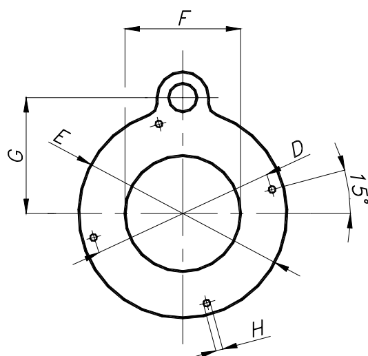
Flange Cosmo 585 - 1200
